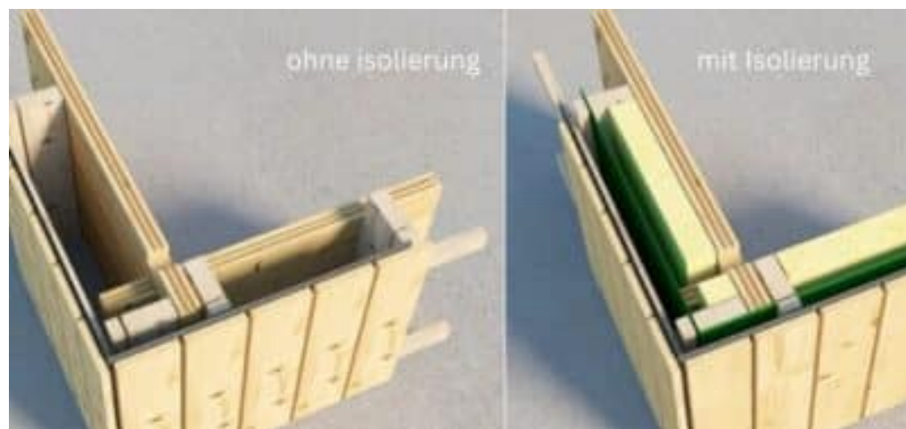
Holzverschalung
